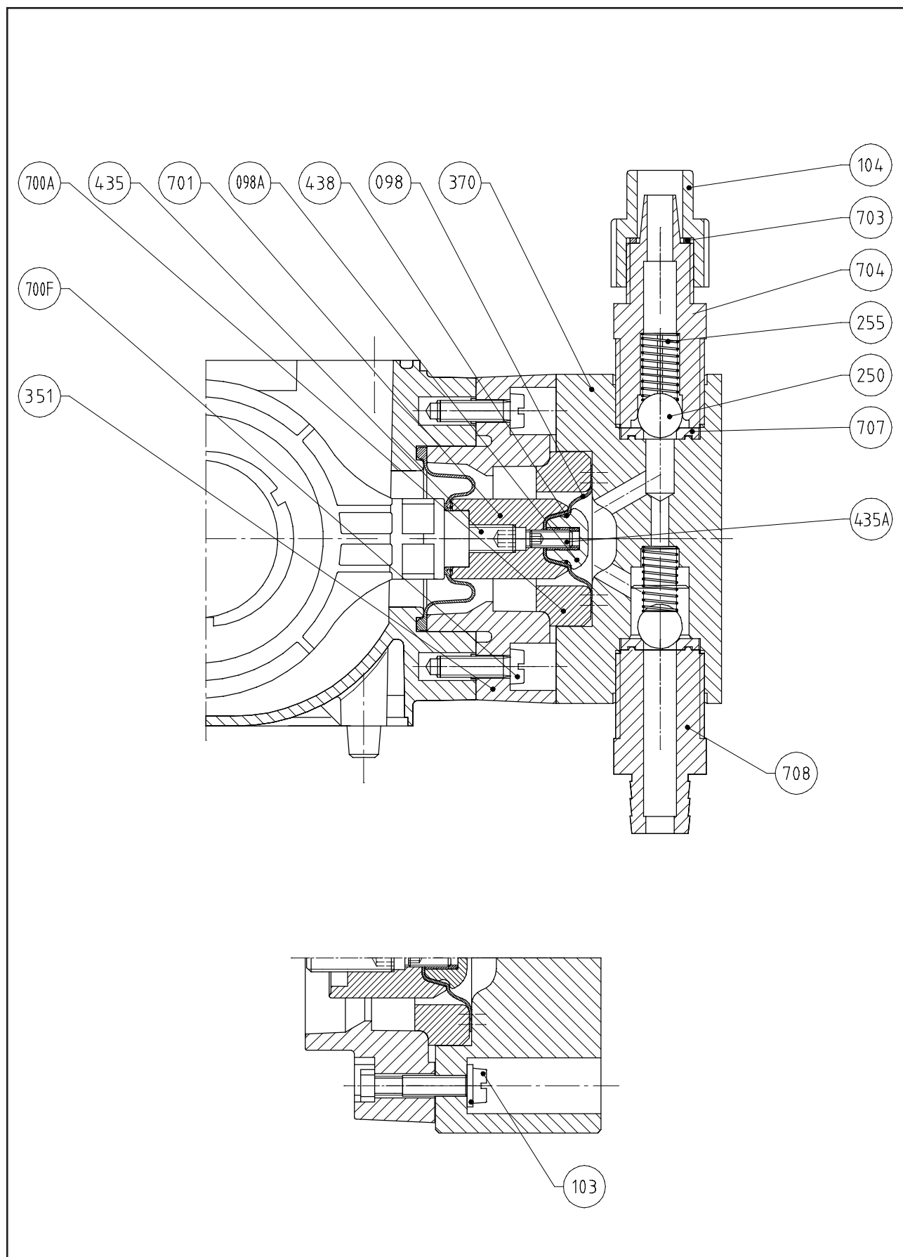
图12 GM0002~GM0010 高粘度液力端
