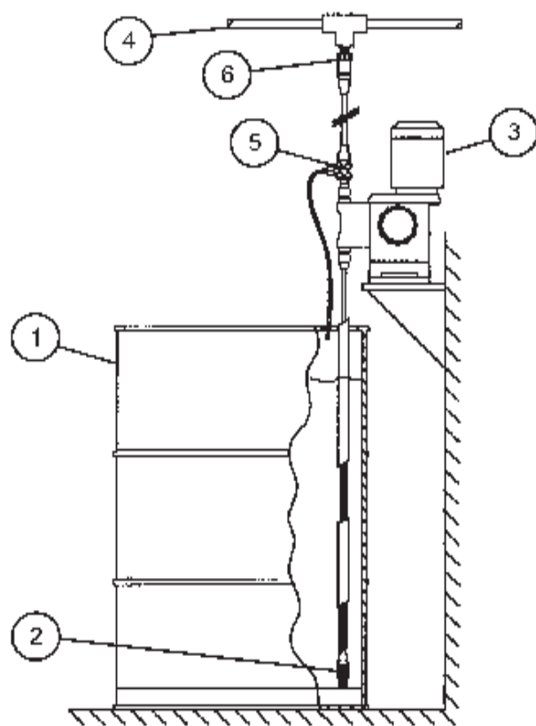
图4: 典型安装
