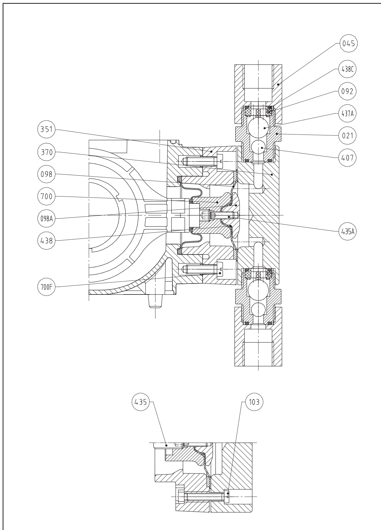
图15 GM0025~GM0050 不锈钢和浆料液力端
