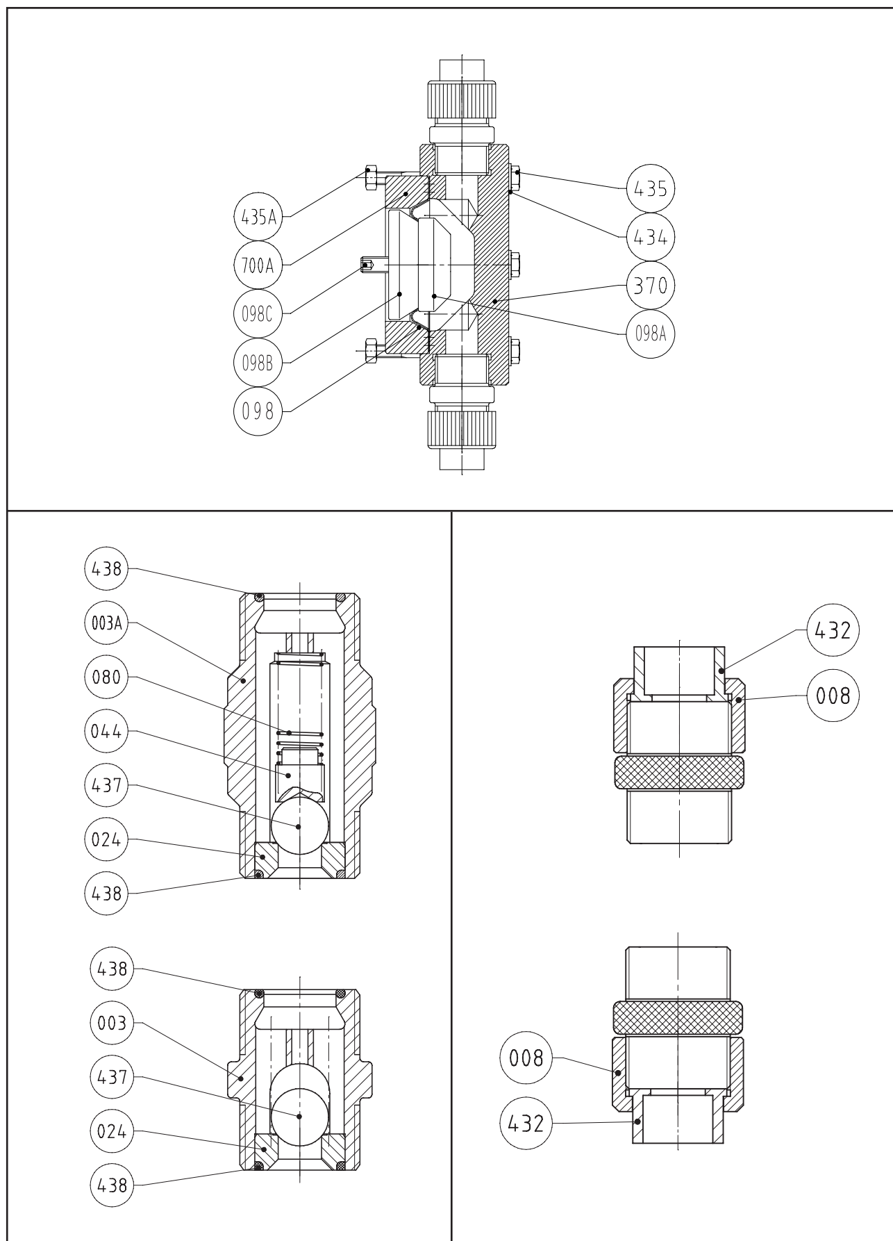
图20 GM0090~GM0500 高粘度液力端
