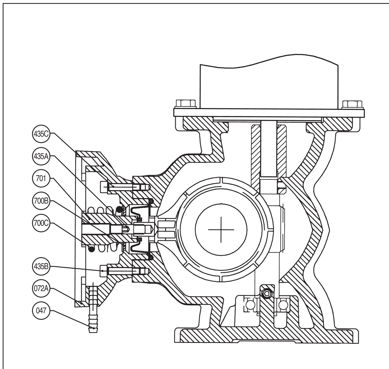
图17 GM0090~GM0500 中间段
