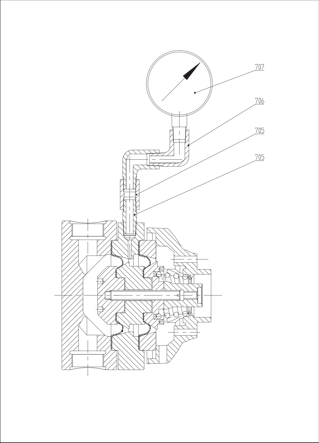
图21 GM双隔膜泵头破裂检测带压力表剖面图
