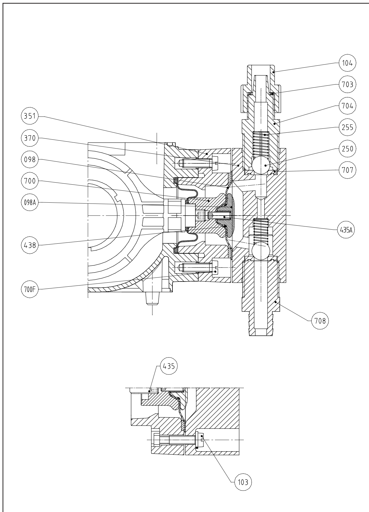
图16 GM0025~GM0050 高粘度液力端
