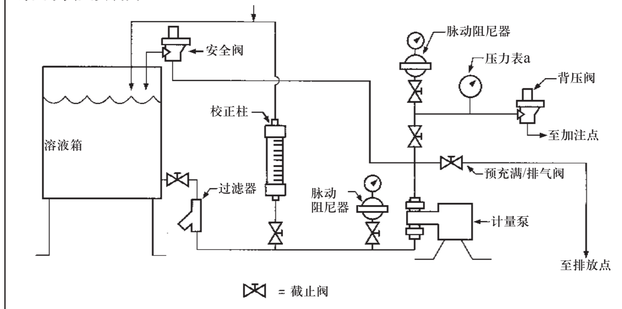
图5: 计量泵典型安装图
