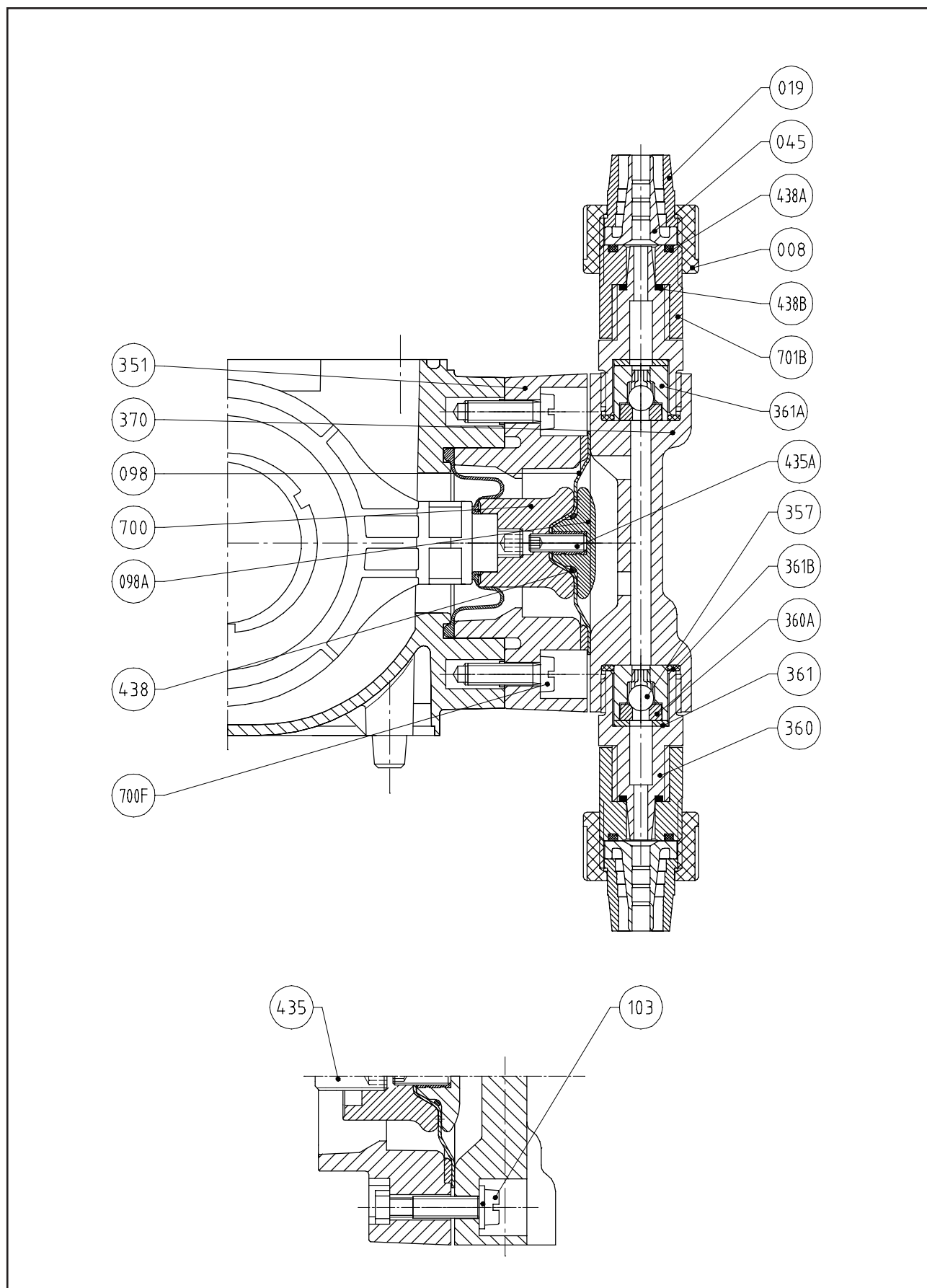
图13 GM0025~GM0050 PVC, PVDF & 混合物液力端
