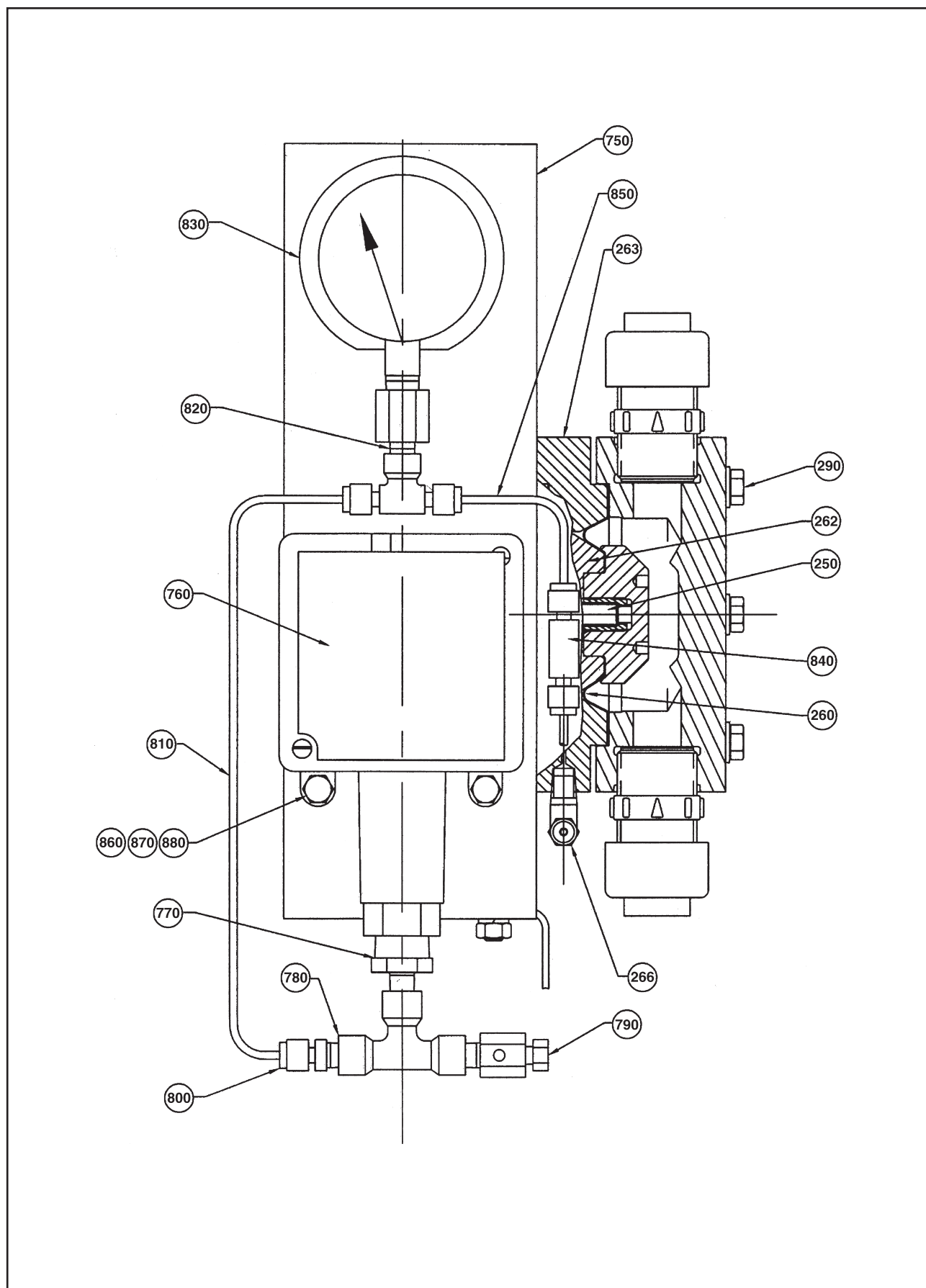
图22 GM双隔膜泵头破裂检测带压力表及压力开关剖面图
