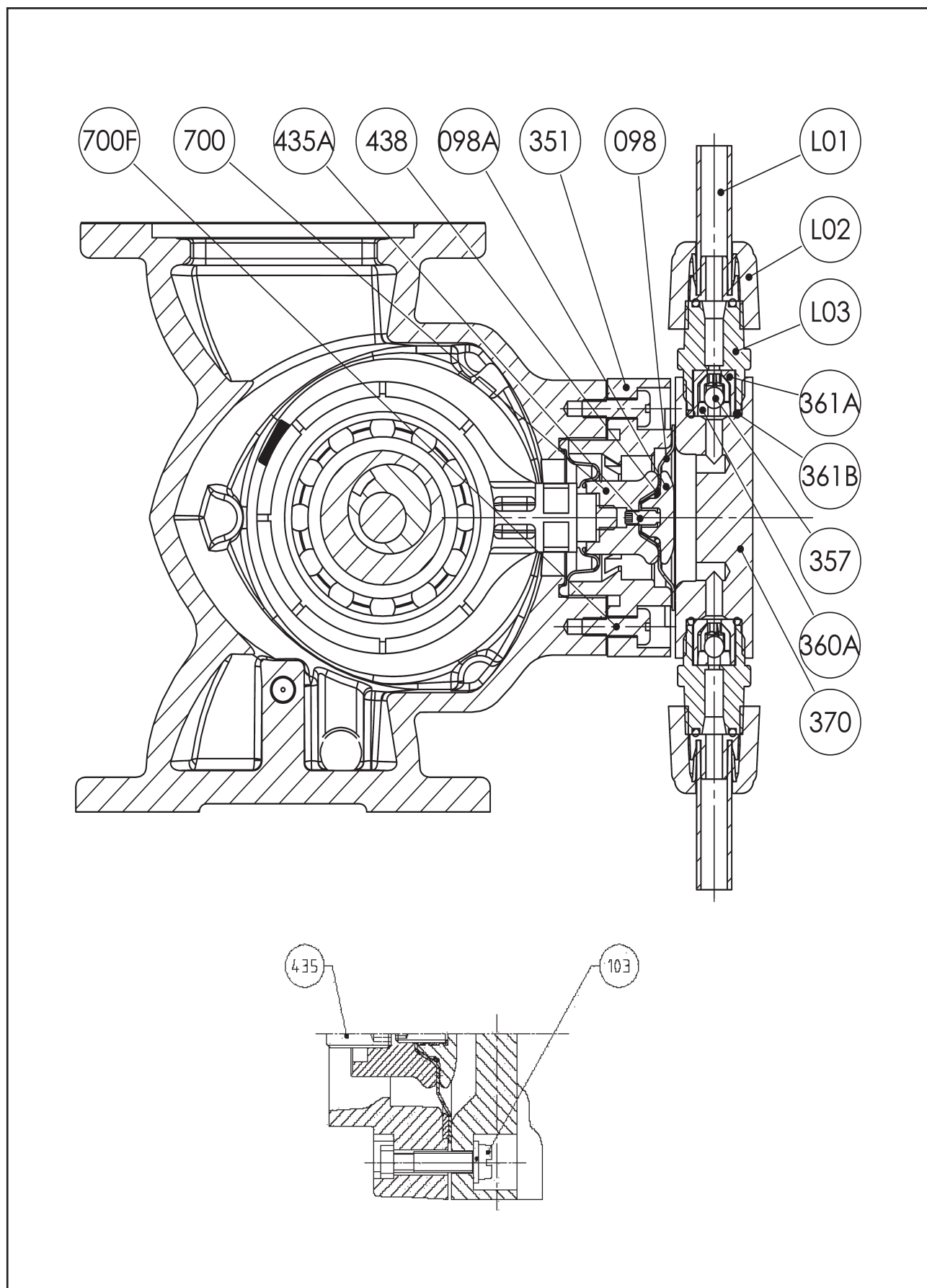
图14 GM0025~GM0050 PVC, PVDF液力端-LMI(PE)软管连接
