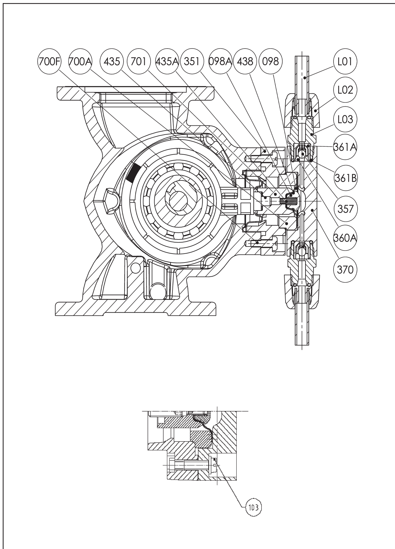
图10 GM0002~GM0010 PVC, PVDF液力端-LMI(PE)软管连接
