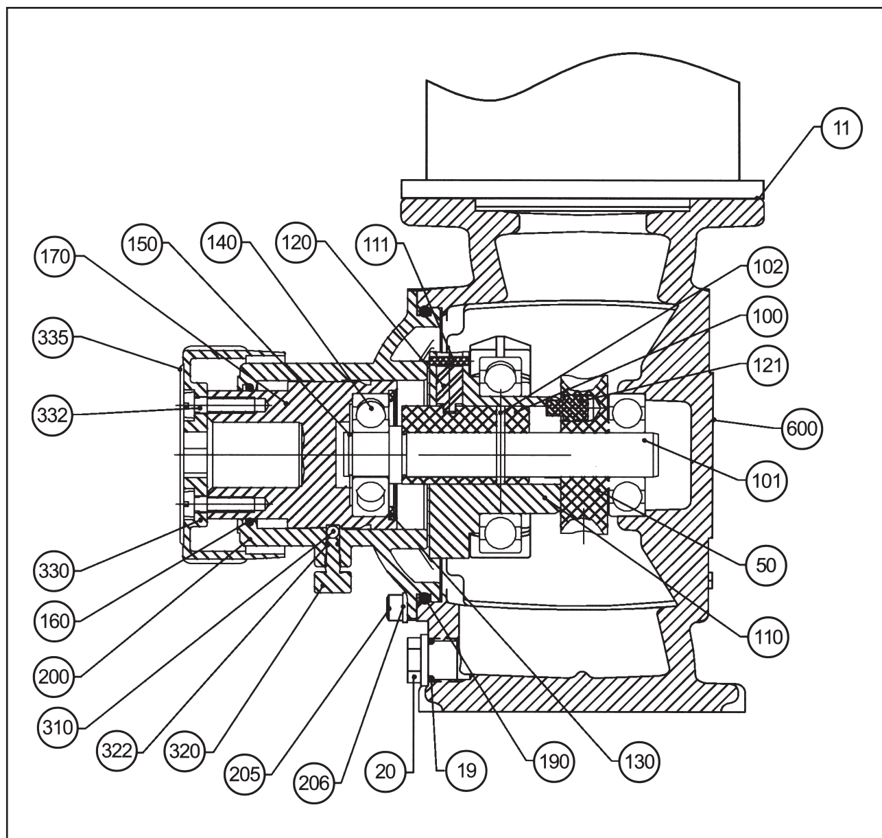
图8 GM 驱动端端面图
